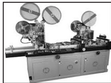
KR545T Tabber
